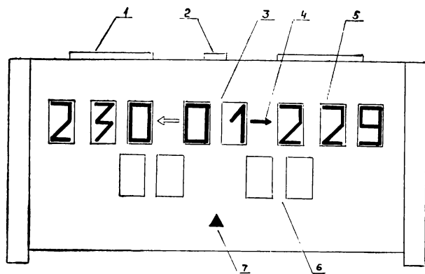
Часы турнирные. 1. Кнопка переключения часов. 2. Кнопка «возврат». 3. Индикатор номера хода. 4. Сигнализатор очередности хода. 5. Индикаторы часов и минут. 6. Индикаторы секунд. 7. Сигнализатор наличия энергии батарей.
