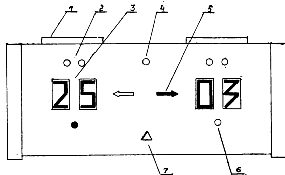
Часы любительские. 1. Кнопка переключения часов. 2. Сигнализаторы остатка времени. 3. Индикаторы минут. 4. Сигнализатор просрочки. 5. Сигнализатор очередности хода. 6. Сигнализатор работы индикаторов. 7. Сигнализатор наличия энергии.
