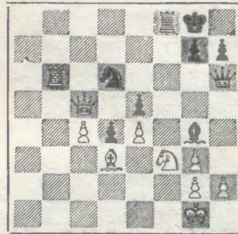
Нафталин
