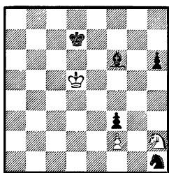
Задача № 1681
