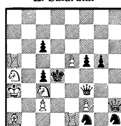
Задача № 1687
