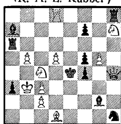
Задача № 1687
