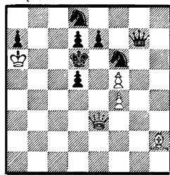
Задача № 1684
