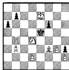
Задача № 1686
