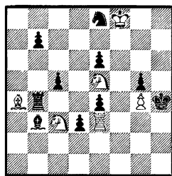
Задача № 1688
