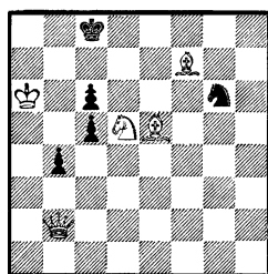
Задача № 1685
