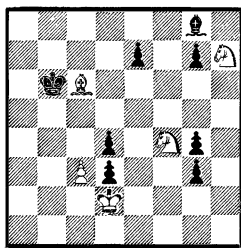
Задача № 1683
