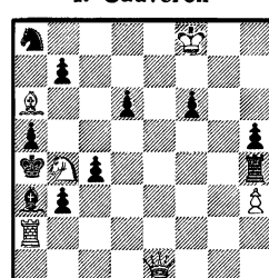
Задача № 1685
