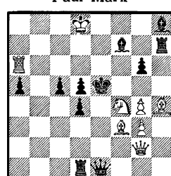
Задача № 1686
