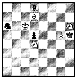
Задача № 1682
