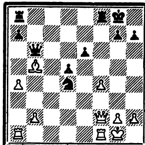
532. Ход черных
