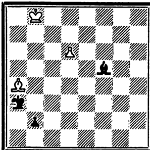
541. Ход белых
