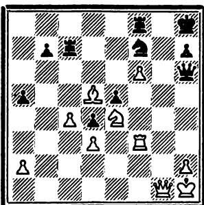
549. Ход белых
