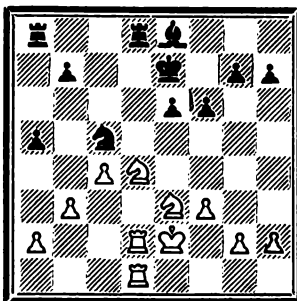
547. Ход белых
