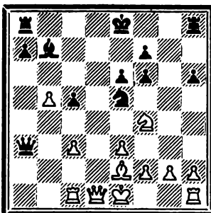
546. Ход черных
