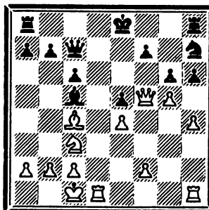
544. Ход белых
