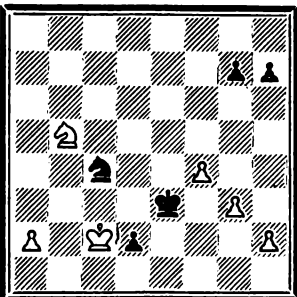
540. Ход черных
