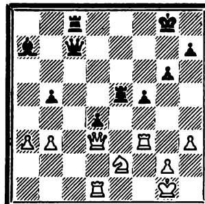
533. Ход черных
