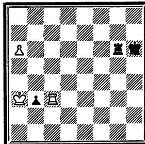
542. Ход белых
