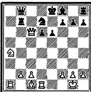
550. Ход белых
