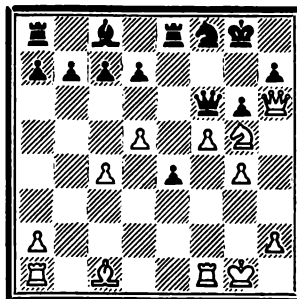
535. Ход белых
