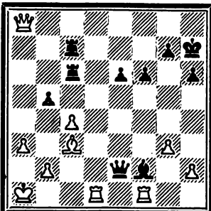
537. Ход черных
