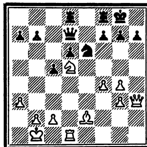
536. Ход белых
