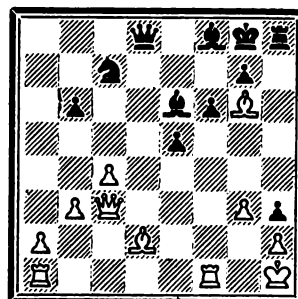
545. Ход черных
