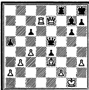
534. Ход белых
