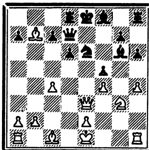
543. Ход белых
