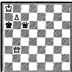
551. Ход белых
