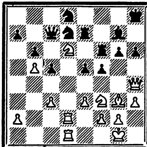
531. Ход белых
