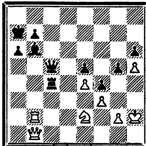
538. Ход черных
